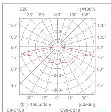
Optika O pre otvorené priestory
